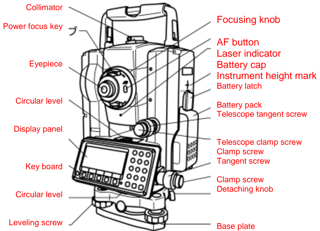
R-325(N)/R-322(N)/R-323(N): Detachable type
